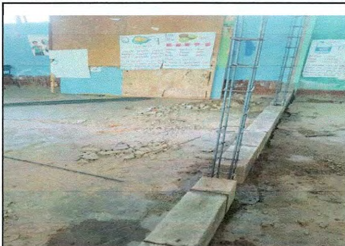
Foto 2: Inicio de colocación de armadura para columnas.
